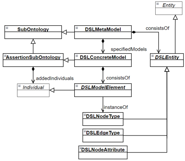
Fig. 6. The model of the pattern for integrating DSLs Рис. 6. Модель паттерна интеграции DSL
