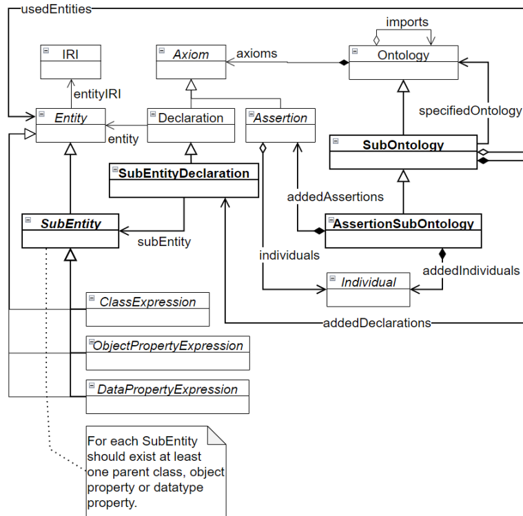
Fig. 5. The model of the pattern for ontology-based metamodeling Рис. 5. Модель паттерна для метамоделирования на основе онтологий
