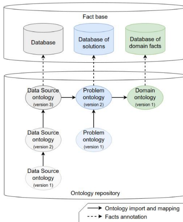
Fig. 2. The basic structure of knowledge base Рис. 2. Базовая структура базы знаний
