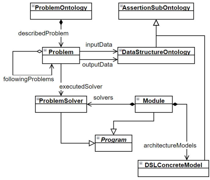
Fig. 7. The model of the pattern for integrating problem solvers Рис. 7. Модель паттерна интеграции решателей
