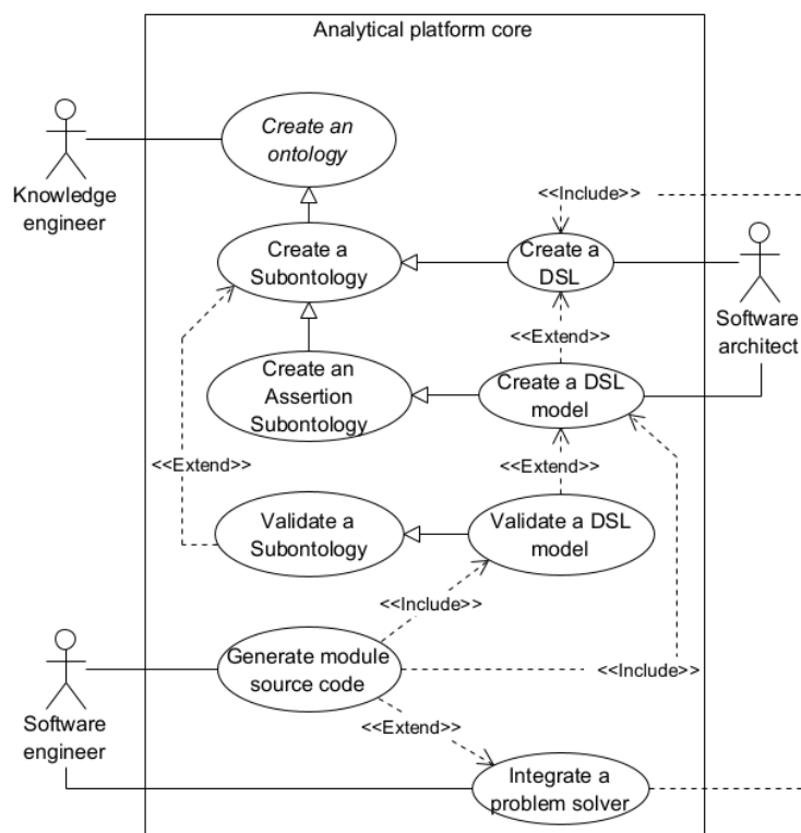
Fig. 9. The functionality of integrating DSLs and problem solvers Рис. 9. Функциональность интеграции DSL и решателей задач
