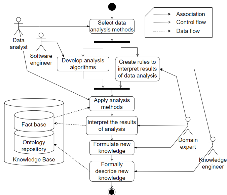
Fig. 1. The model of process of data analysis and interpretation Рис. 1. Модель процесса анализа и интерпретации данных
