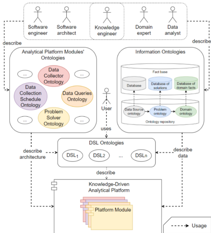
Fig. 3. An approach to analytical platform development Рис. 3. Подход к разработке аналитической платформы
