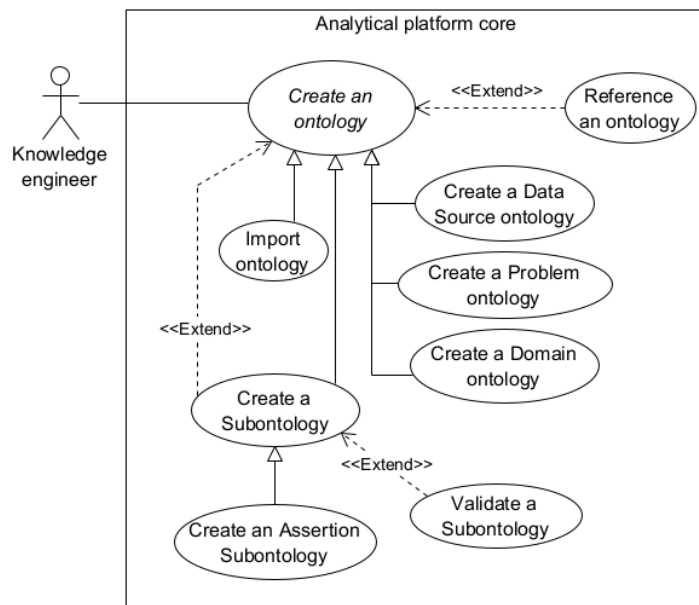
Fig. 8. The functionality of the tools for managing the repository of ontologies Рис. 8. Функциональность средств управления репозиторием онтологий
