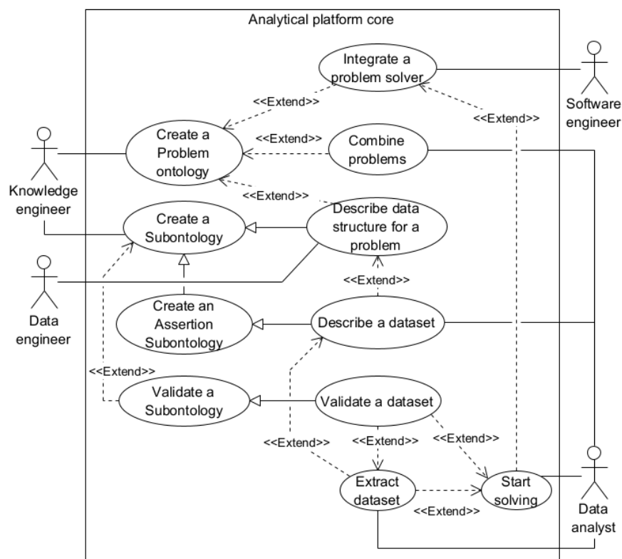
Fig. 10. The functionality of managing problem solving Рис. 10. Функциональность управления решением задач
